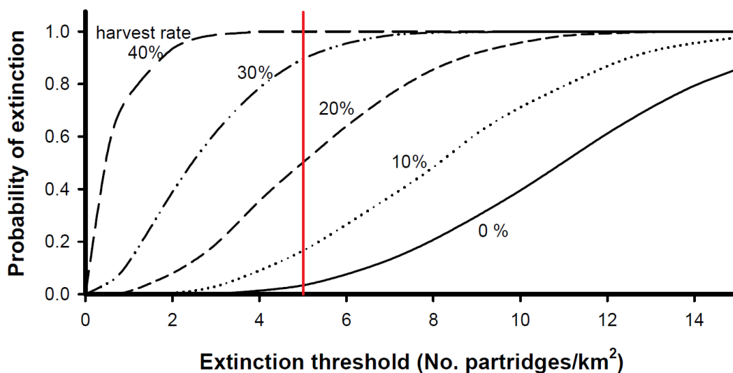
Figuur 12: Kans op uitsterven onder 5 verschillende jachtintensiteiten (harvest rate) in functie van verschillende drempelwaarden voor de voorjaarsdensiteit (extinction threshold) volgens het populatiemodel van De Leo et al. (2004) op basis van populatiekenmerken van Frankrijk, Polen en Italië. De drempelwaarde van 5 patrijzen per km² is aangeduid in het rood en vormt volgens de auteurs een realistische drempelwaarde waaronder gefragmenteerde populaties kunnen uitsterven. Uit De Leo et al. (2004).
